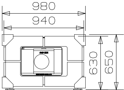
Front@1
